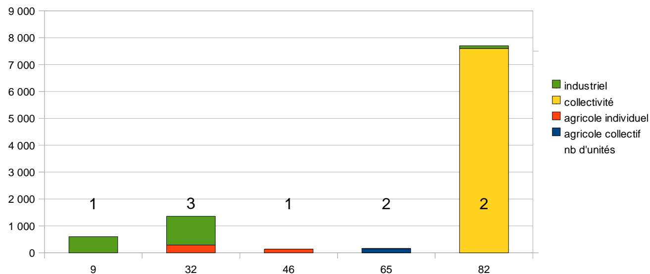
Unités de cogénération en service en Midi-Pyrénées au 15/06/2014, données DRAAF-DDT-DREAL
